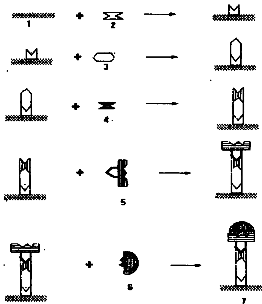
Рисунок 3. Схематическое изображение "сэндвич"-варианта иммуноферментного анализа антител.
