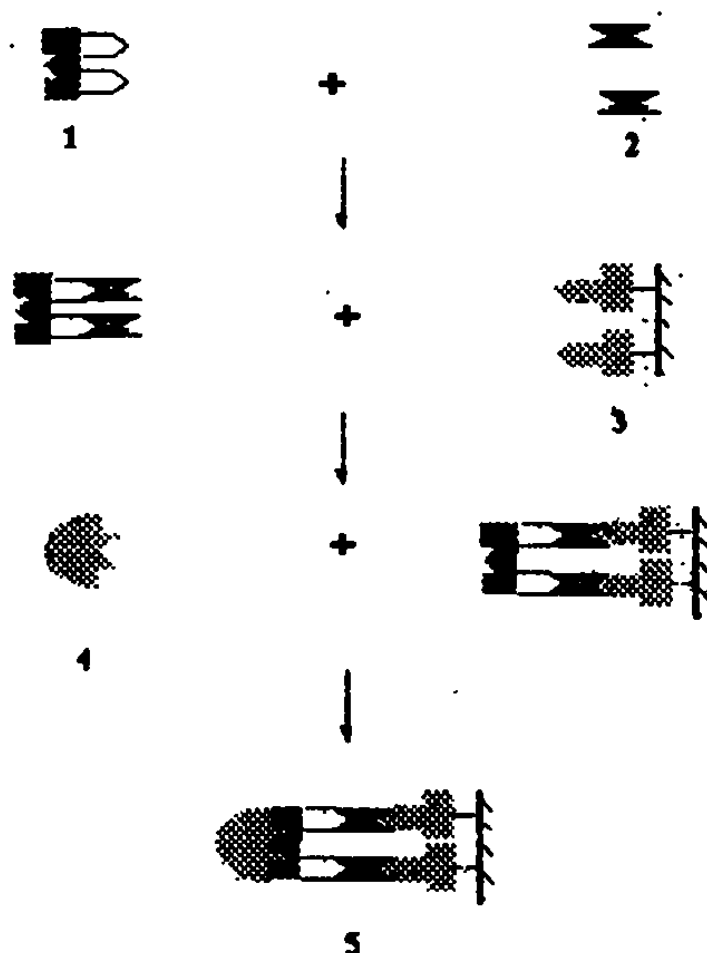
Рисунок 4. Схематическое изображение двухцентрового варианта иммуноферментного анализа
